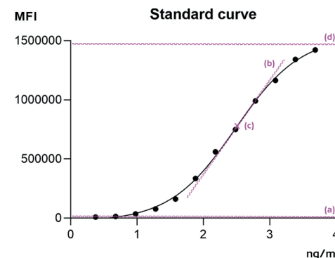
Figura 5: Curva de forma sigmoidea correspondiente a la ecuación del modelo de regresión logística de cuatro parámetros (4PL).
